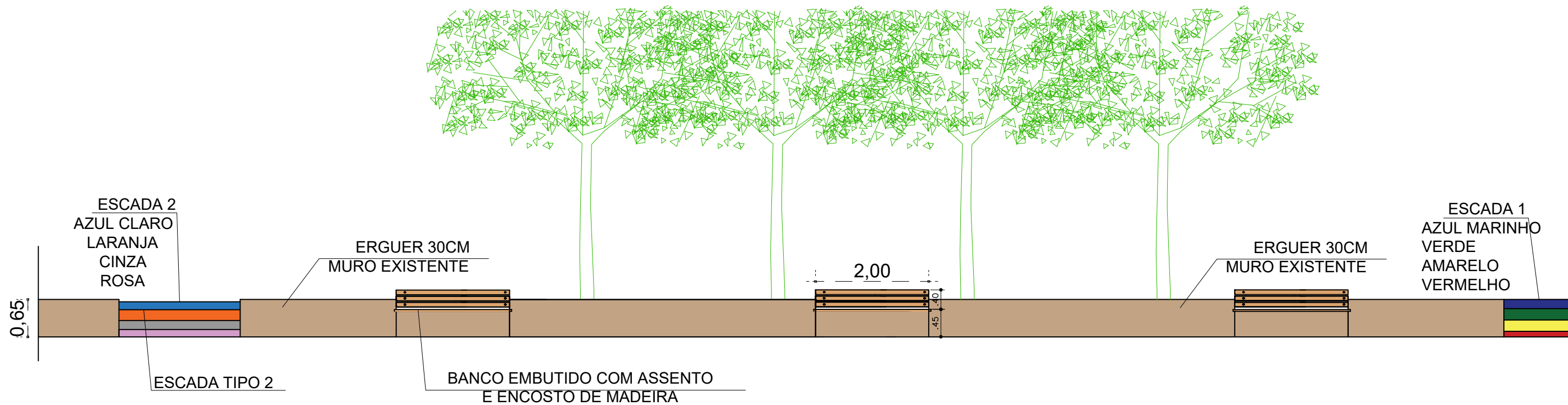
3 CANTEIRO 2 - VISTA LONGITUDINAL ESC. 1/75
