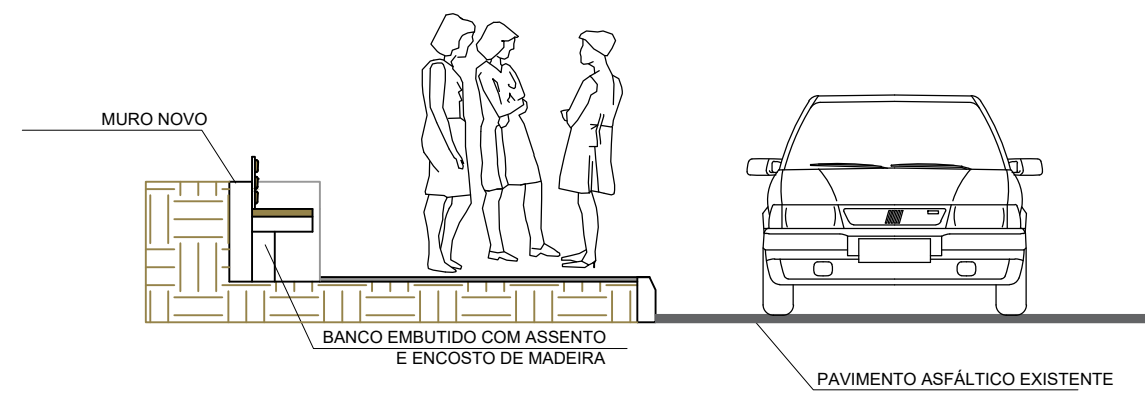
4 PERFIL TRANSVERSAL ESC. 1/50
